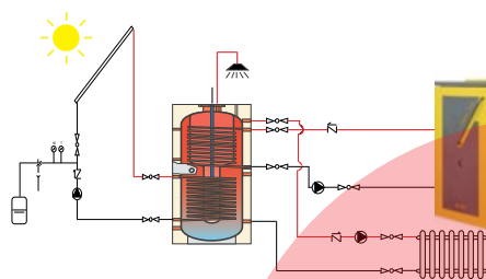
Συνδεσμολογία με μπόιλερ tank in tank, ηλιακούς συλλέκτες
