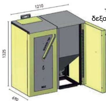
Νέος πυρολυτικός καυστήρας
