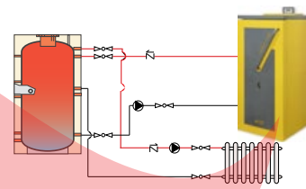
Συνδεσμολογία με μπόιλερ buffer
