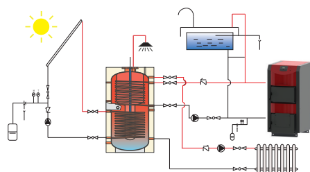
Συνδεσμολογία με μπόιλερ tank in tank , ηλιακούς συλλέκτες και ανοιχτό δοχείο διαστολής
