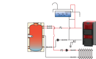
Συνδεσμολογία με μπόιλερ buffer
